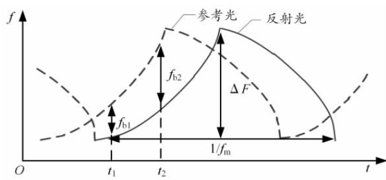
图 1 光源扫频非线性效应示意图
