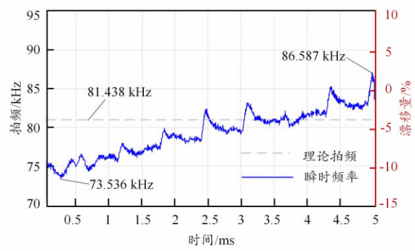
图 2 附加干涉仪拍频信号频率及偏移量
